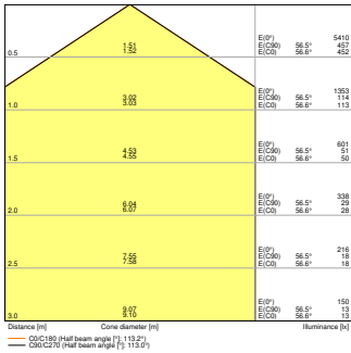
PL CMFT 600 P 33W 830 PS EM
