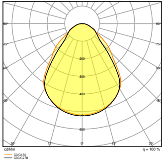
PL CMFT 600 P 33W 830 U19 DALIVR
