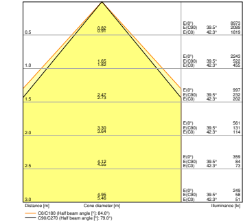
PL CMFT 600 P 33W 830 U19 PS
