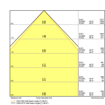
PL CMFT 600 P 28W 830 U19 PS
