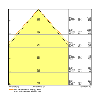
PL CMFT 600 P 30W 830 U19 PS
