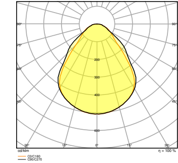
PL CMFT 600 P 28W 830 U19 PS
