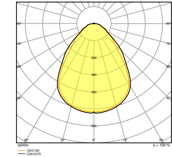
PL CMFT 600 P 33W 830 U19 PS EM CONVERSION BOX
