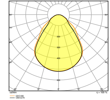
PL CMFT 600 P 30W 830 U19 PS
