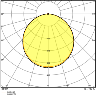
PL CMFT 600 P 33W 830 PS EM CONVERSION BOX
